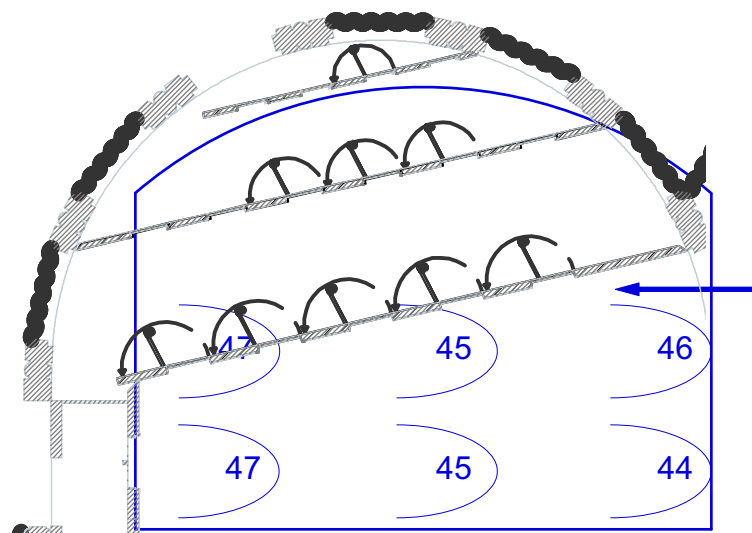
SL Sidelight B (2 units per lane)
